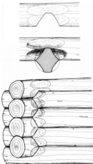
L'entaille en « tête de Bœuf »
